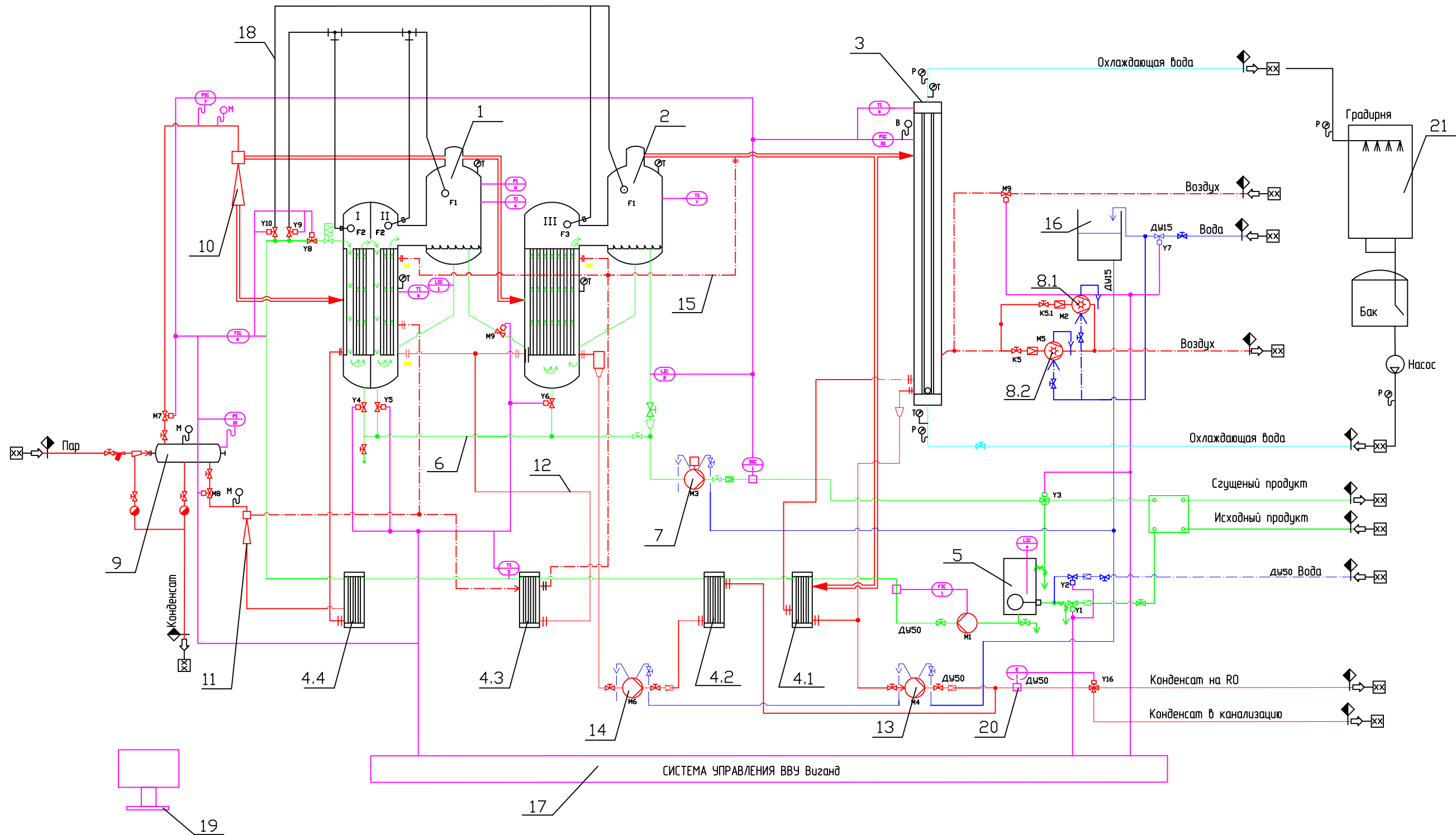
ПРИНЦИПАЛЬНАЯ СХЕМА модернизированной ВВУ Vizand 8000
